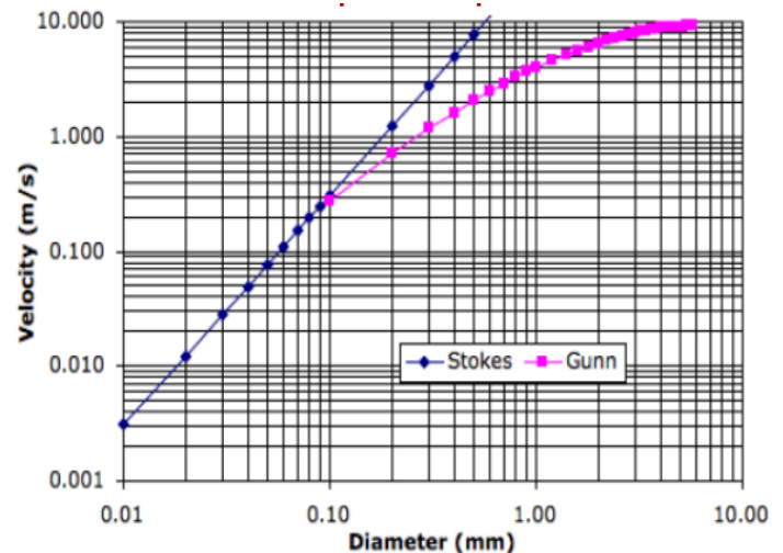
Fig 6 curva caratteristica separazione sabbie in funzione della granulometria
