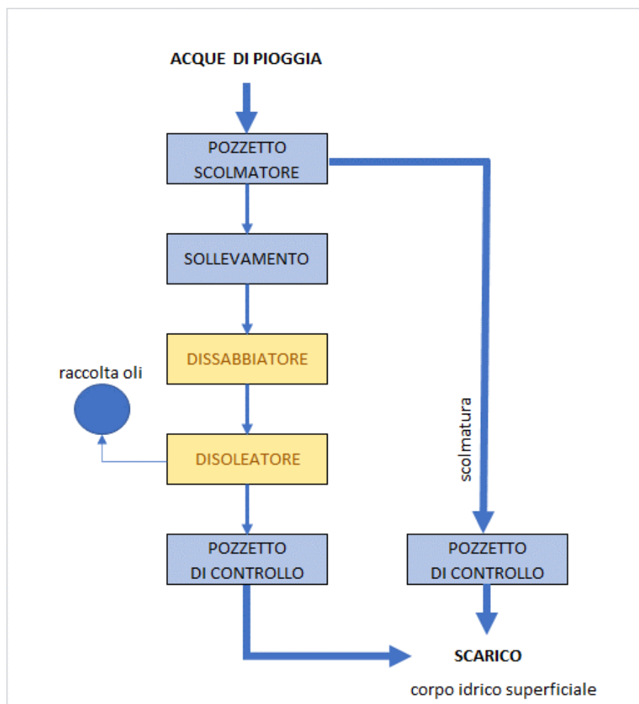
Fig 3 Schema a Blocchi
