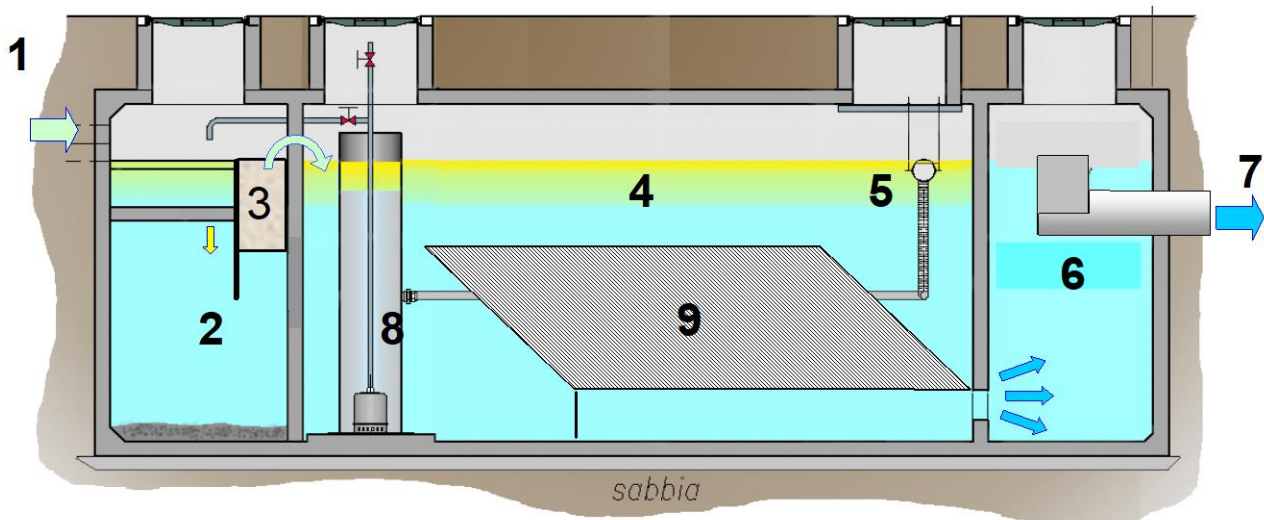
Fig.5 - 1. acque di pioggia in arrivo, 2. dissabbiatore, 3. ev. coalescer, 4. zona affioramento oli, 5. raccogliore oli, 6. vasca effluente depurata, 7. acque trattate allo scarico, 8. raccogliore olio pompa livellatrice svuotamento, 9. pacco lamellare.
