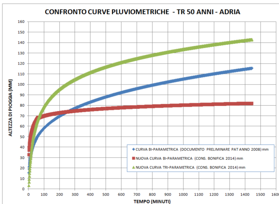
FIG. 02 – CONFRONTO CURVE PLUVIOMETRICHE
